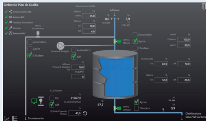
Tlo vèijen la situazion dl resservar sun Plan de Galba, tan de ega che ruva ite (5,9 lt/sec.), tanta che n va ora (0,9 lt/sec.) y tan plèn che l'ie. Te chèsc resservar iel ntegrà n sistem automatic a UV per garanti for na ega nèta.
